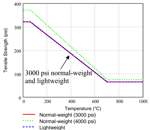
(d) Tensile strength
