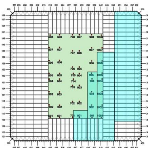
(d) Floor 82
